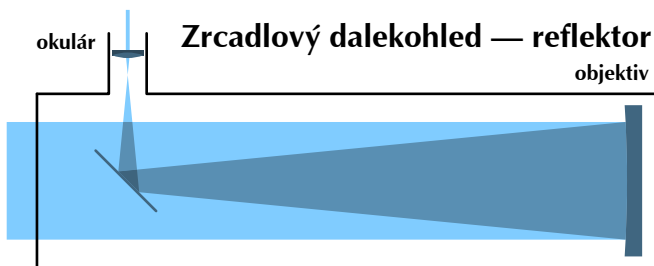
Zrcadlový dalekohled
