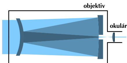
Katadioptrický dalekohled
